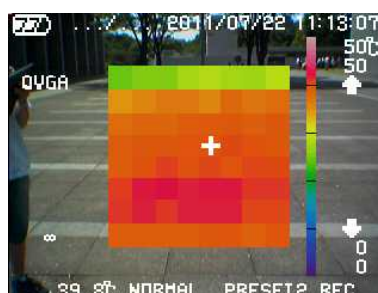
放水前の地面の温度分布
